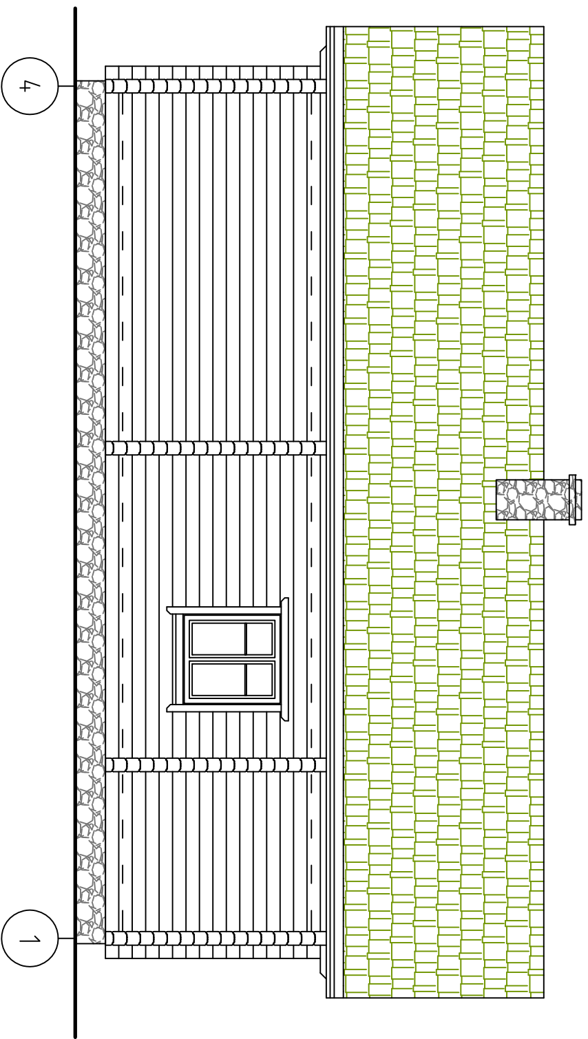
Фасад в осях "4" - "1"
