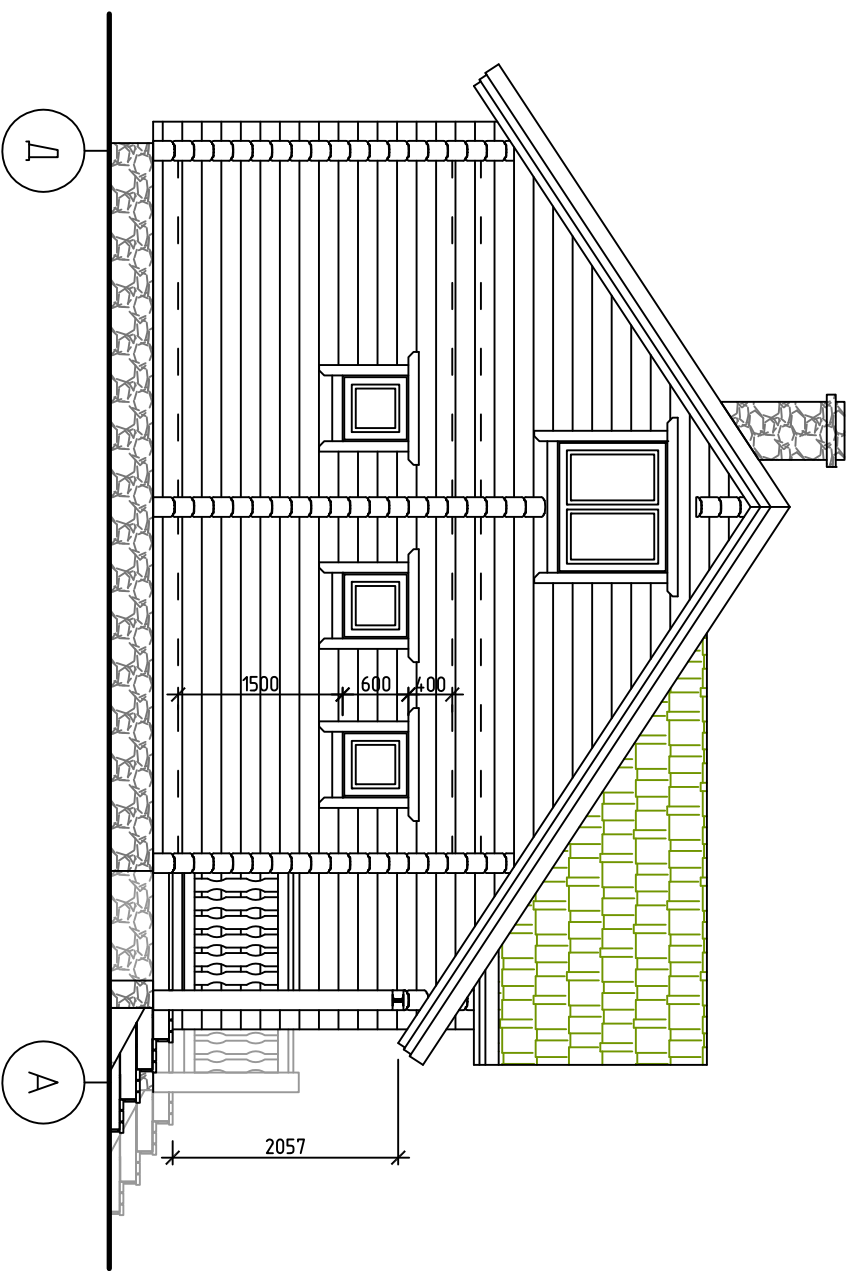
Фасад в осях "Д" - "А"
