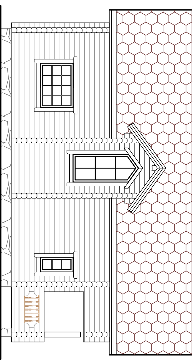
ФАСАД В ОСЯХ "А" – "Ж"
