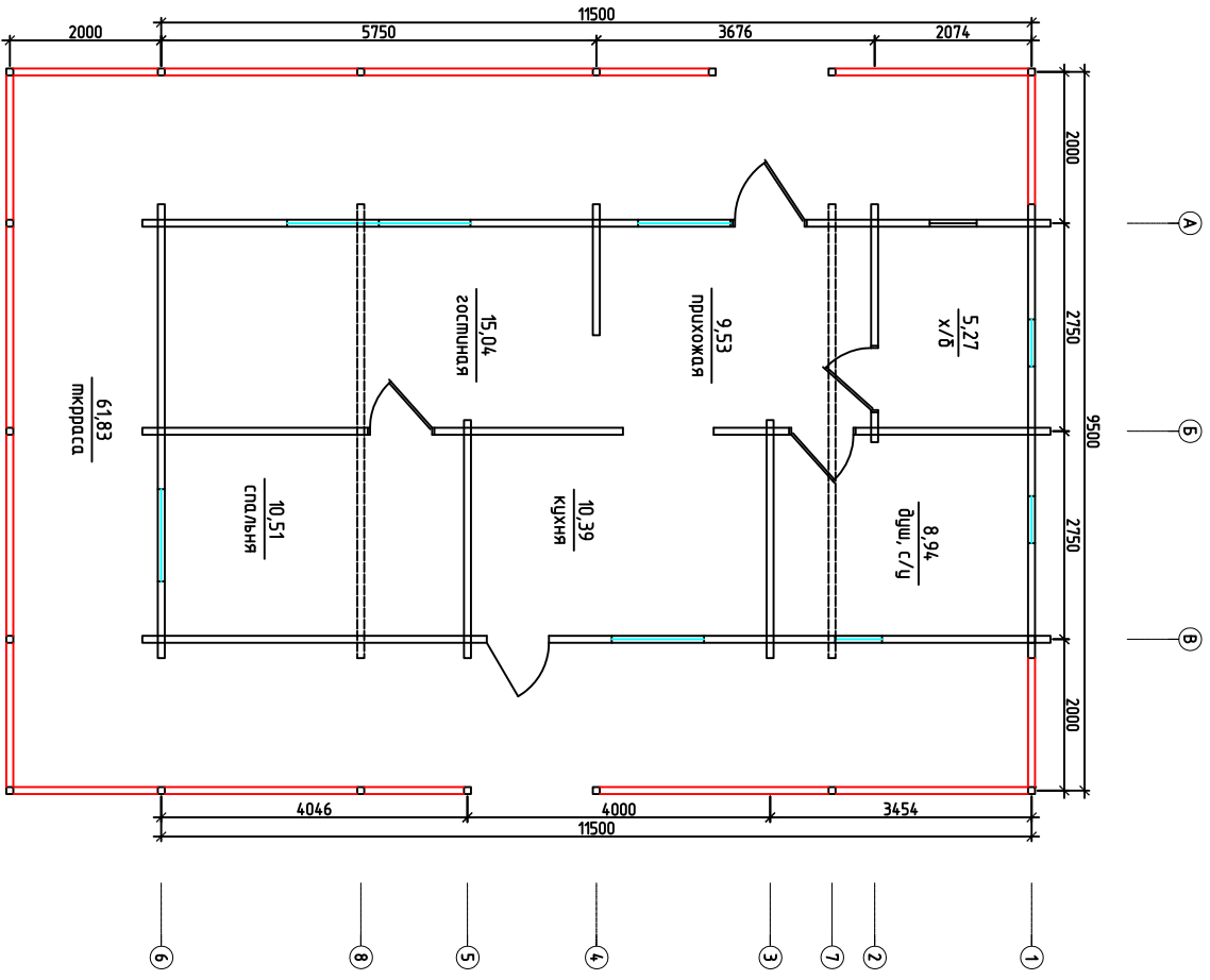
План первого этажа
