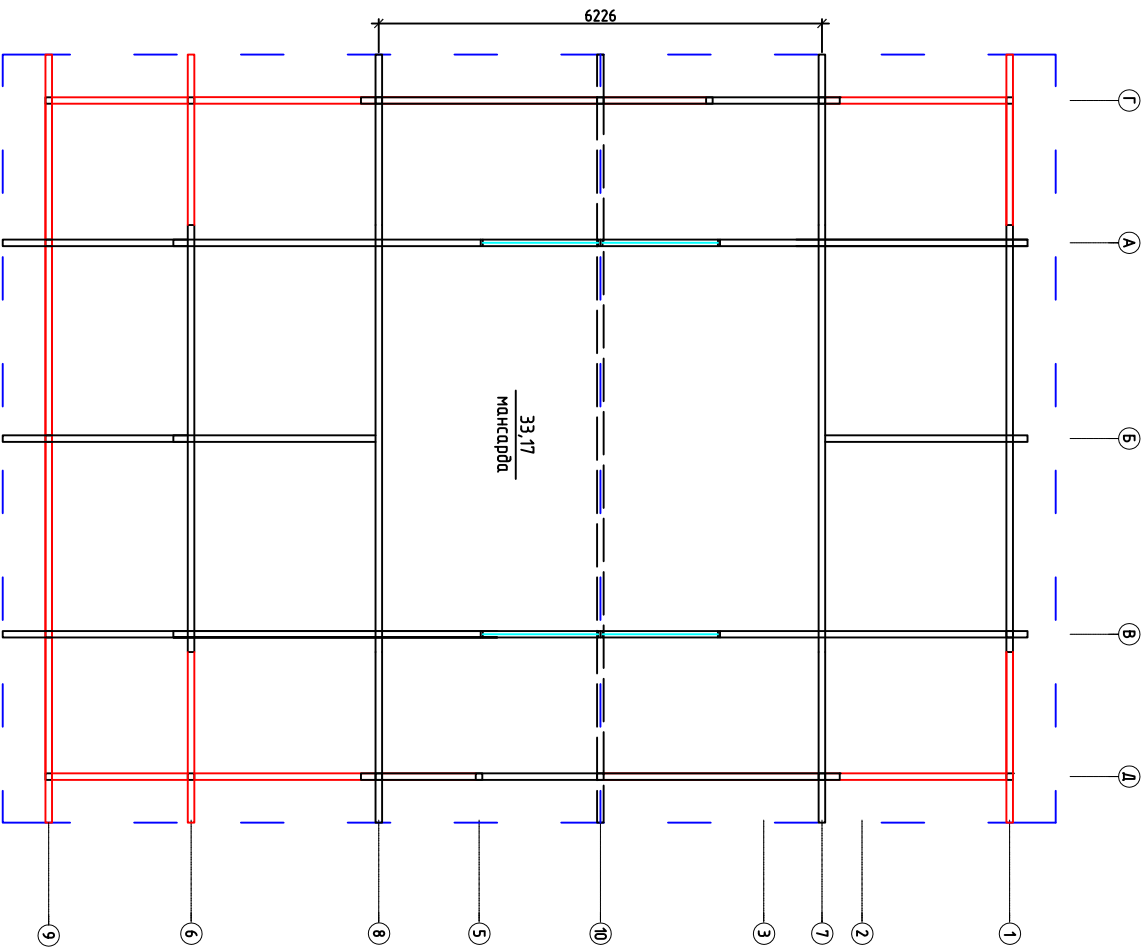
План второго этажа
