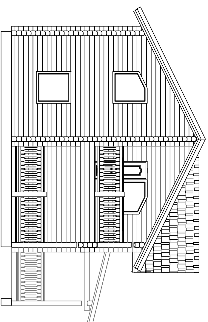
Фасади по осу Г
