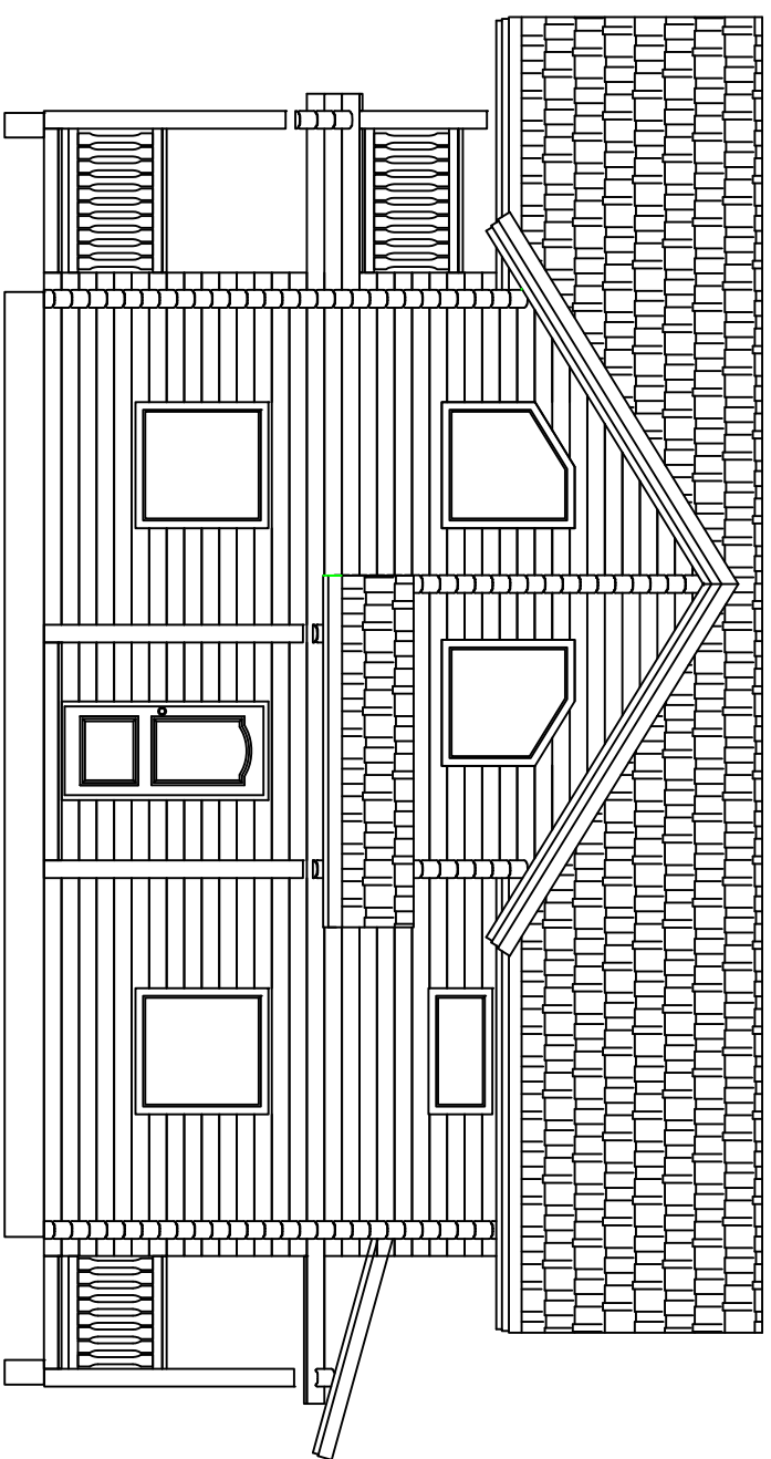
Фасади по осу А
