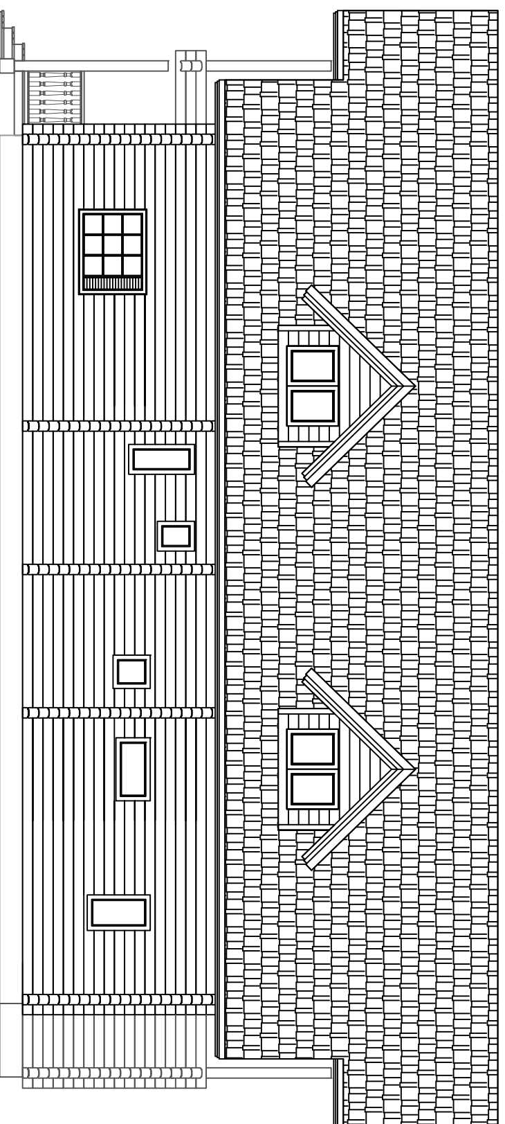
Фасади по осу 1; 2
