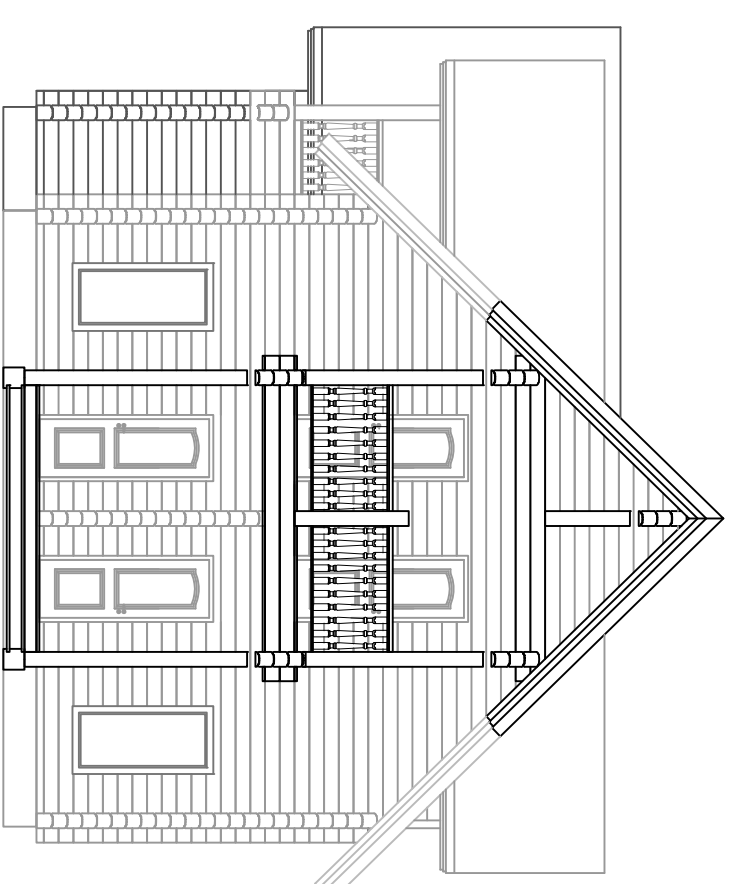
Фасади по осу А; В; Е
