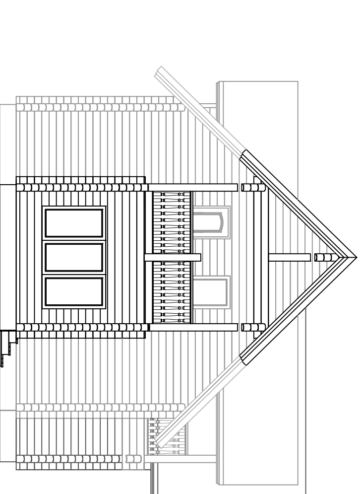
Фасади по осу И; К; Л; М
