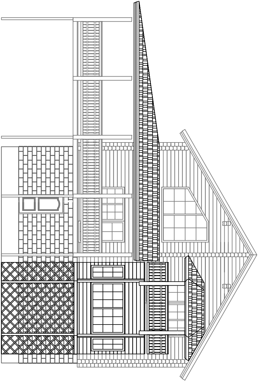
Фасад по оси В
