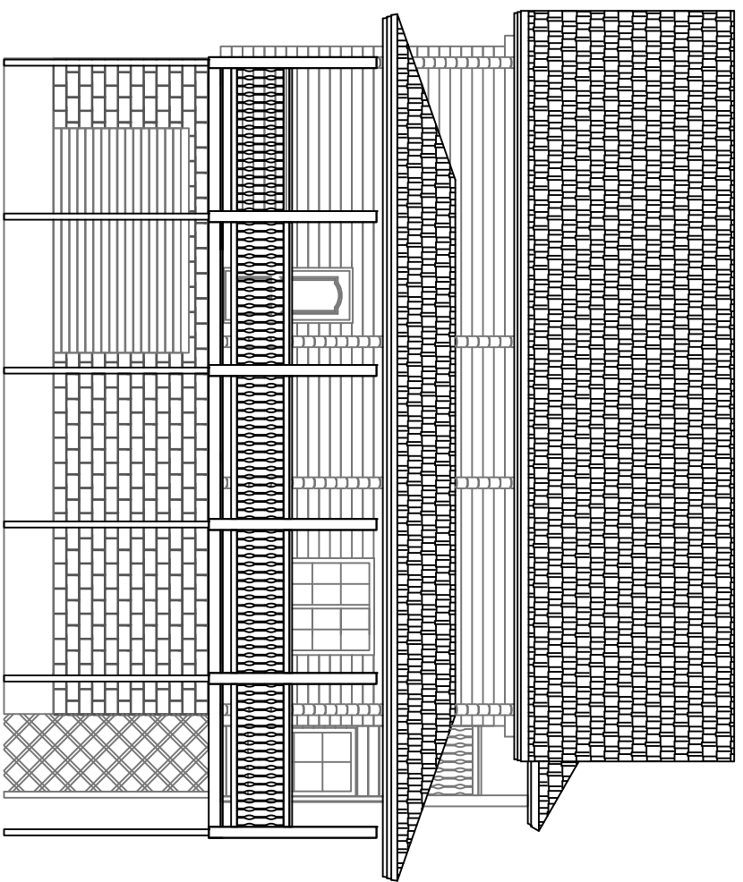
Фасад по оси 2
