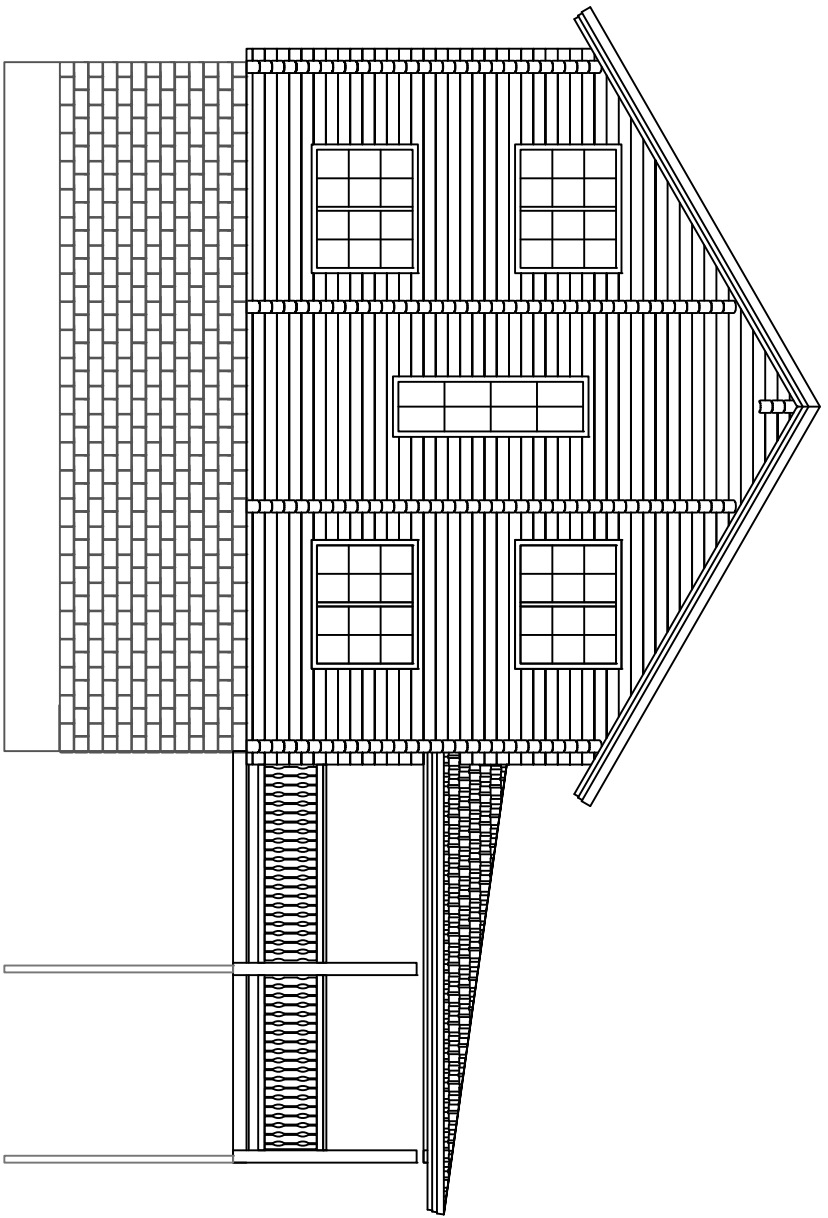
Фасад по оси Ж
