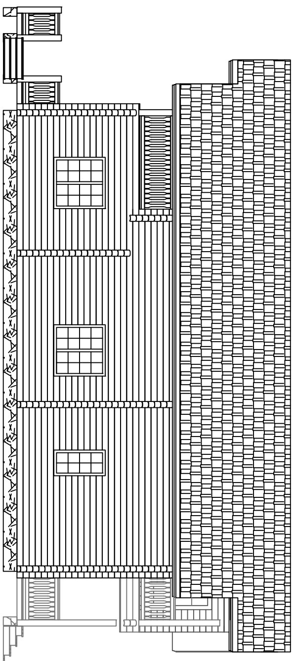
Фасада по осу 5
